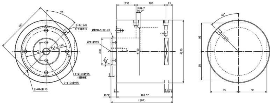
CUREX用加圧シリンダ
