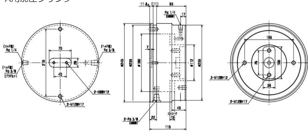
CUREX用加圧シリンダ
